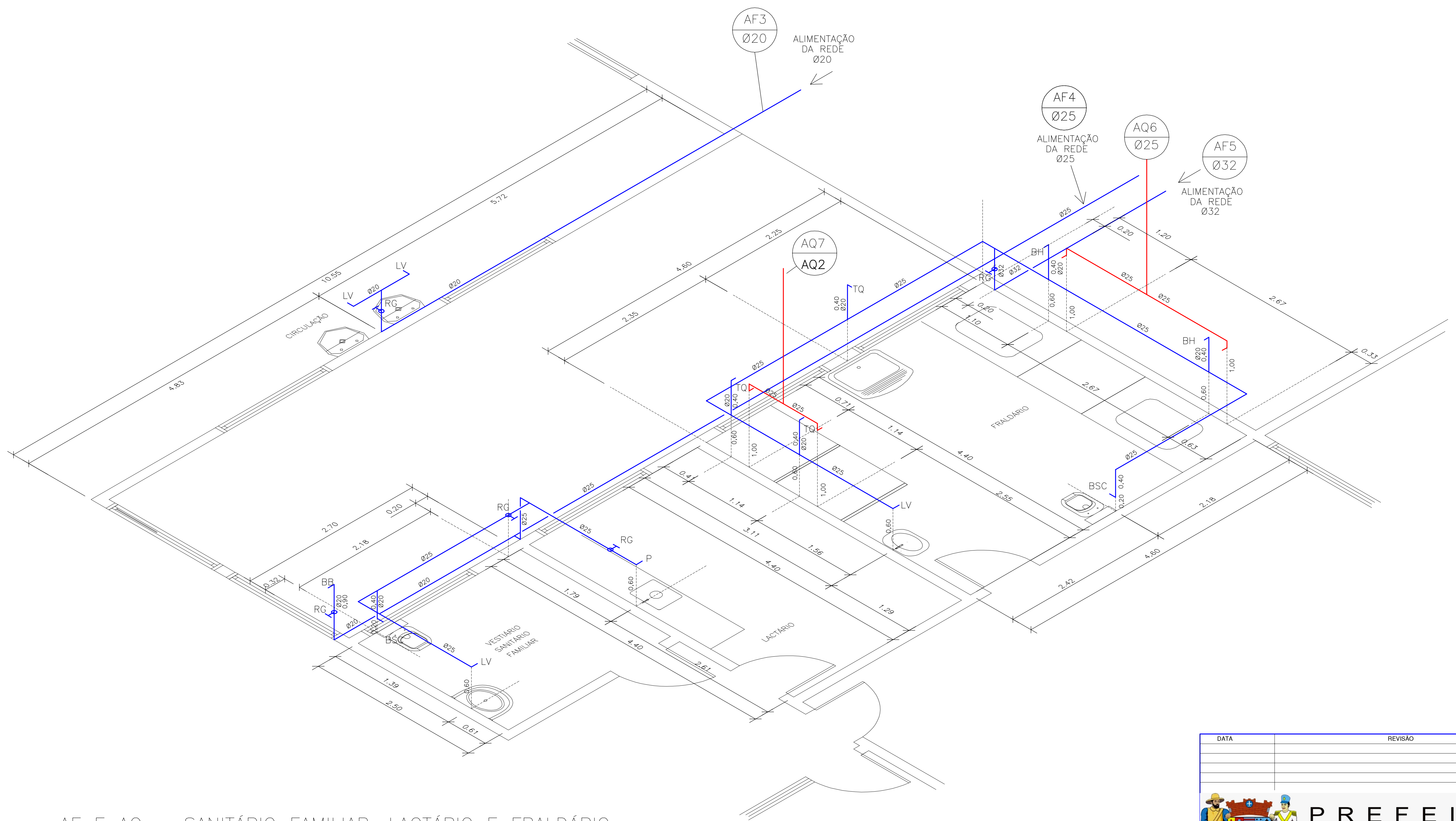
AF E AQ – SANITÁRIO FAMILIAR, LACTÁRIO E FRALDÁRIO E CIRCULAÇÃO esc.: 1:50
